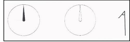
شكل رقم(4) العدد الهندسي واحد (زاوية واحدة)
