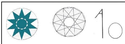
شكل رقم(9) العدد الهندسي عشرة (عشر زوايا)
